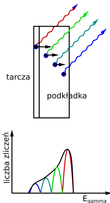
Rys. ŚLCJ-7.13: Pomiar czasu życia metodą DSAM. Kolorem czerwonym oznaczono kwanty gamma emitowane w locie, przy pełnej prędkości emitującego jądra. Kolor niebieski oznacza kwanty emitowane w spoczynku, a zielony – przy pośrednich prędkościach (rys. M.Zielińska)
