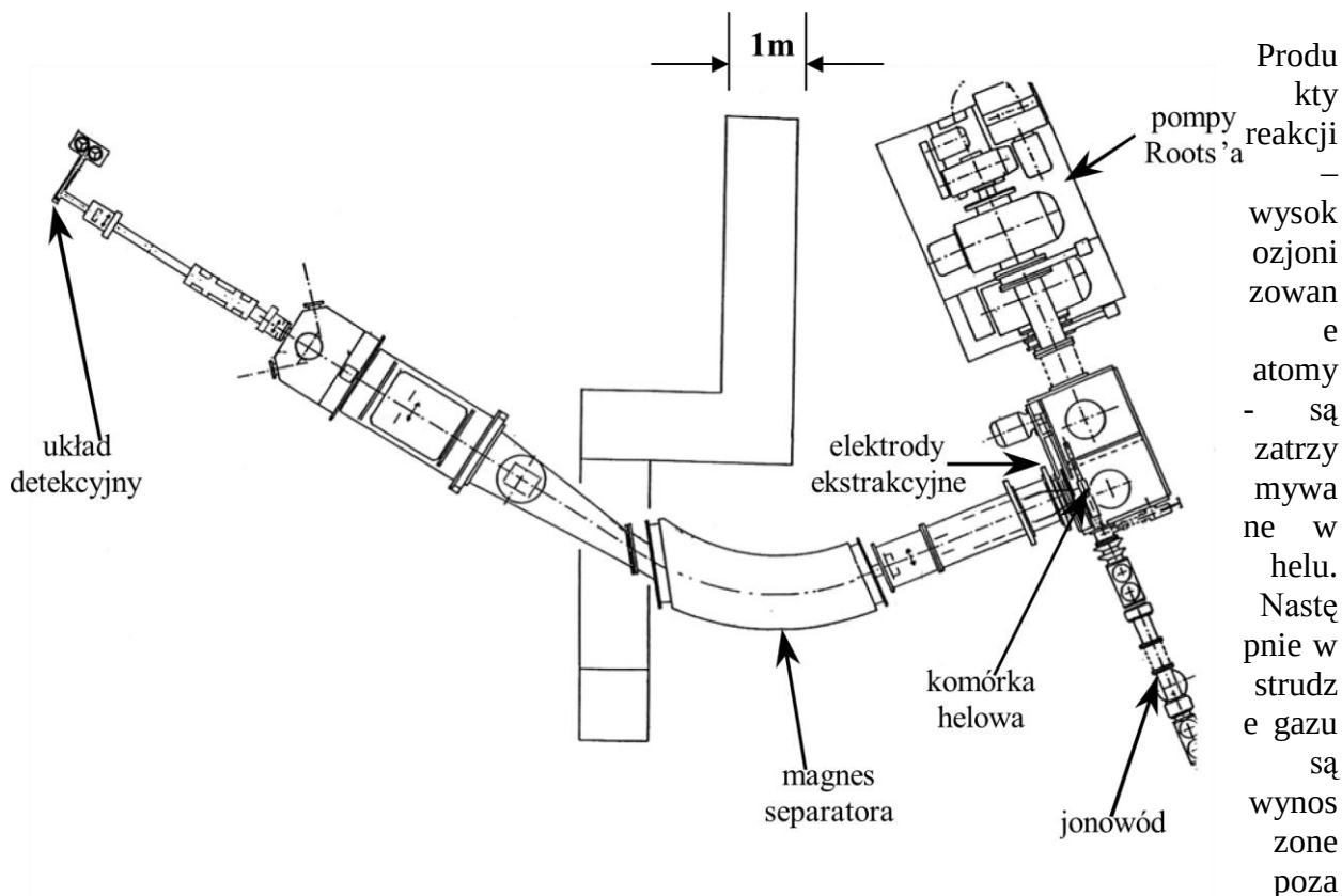
Rys. ŚLCJ-7.14: Schemat układu WIGISOL (rys. z pracy magisterskiej O.Steczkiwicz)
