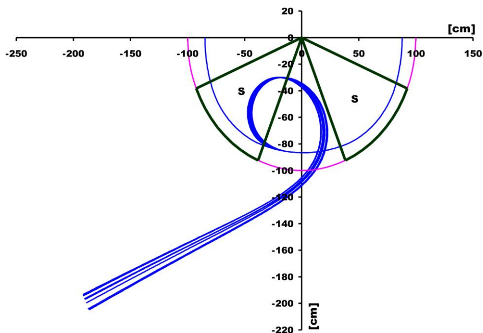
Rys. ŚLCJ-7.5: Wyprowadzenie jonów ^{14}\text{N}^{+3} przez zmianę ładunku do stanu 7+ , z promienia 83 cm. Literami „s” zaznaczono sektory, czyli obszary o wyższym polu magnetycznym (rys. J. Choiński)
