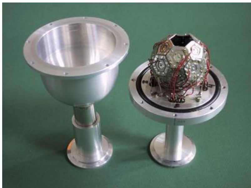
Rys. ŚLCJ-7.9: SiBall - układ detektorów krzemowych do rejestracji i identyfikacji protonów i cząstek alfa w koincydencji z detektorami germanowymi układu EAGLE (fot. A. Kordyasz)
