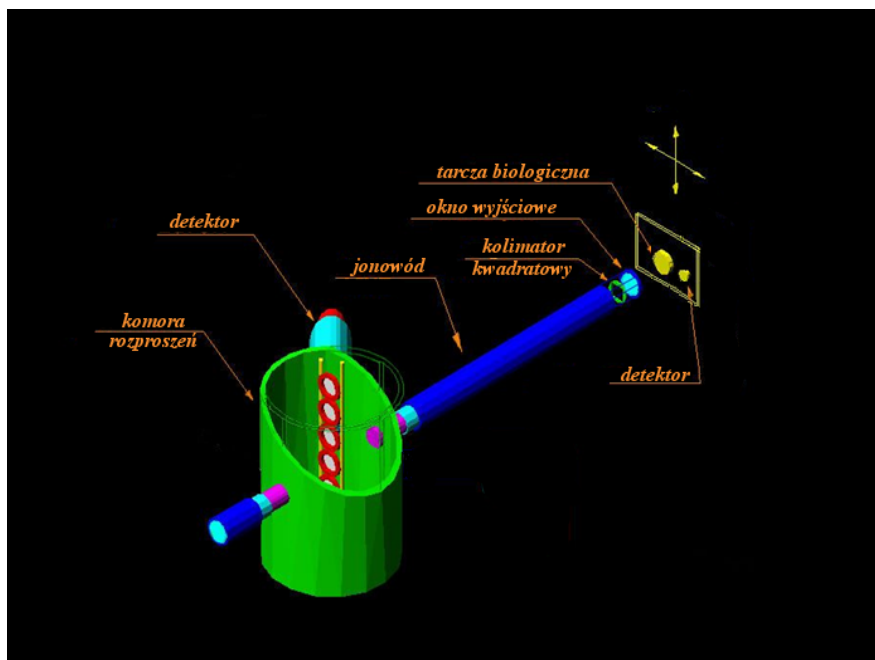
Rys. ŚLCJ-7.20: Schemat układu pomiarowego do badań radiobiologicznych (rys. Z.Szepliński).
