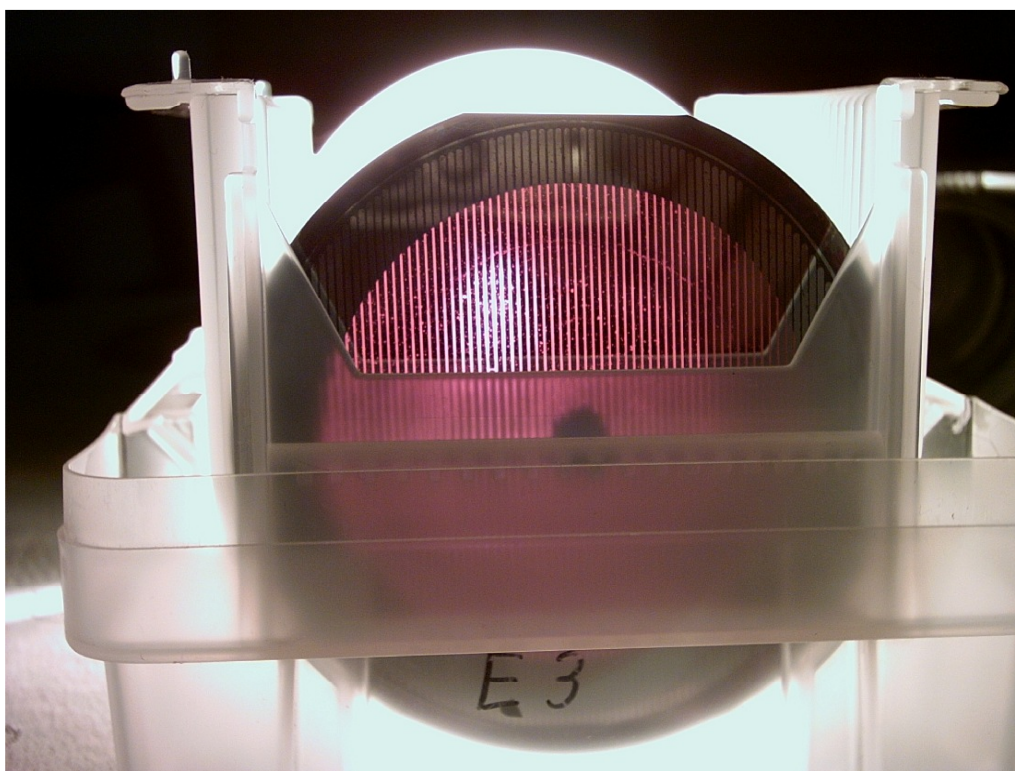
Rys. ŚLCJ-7.22: Krzemowy detektor paskowy zbudowany w ŚLCJ.
