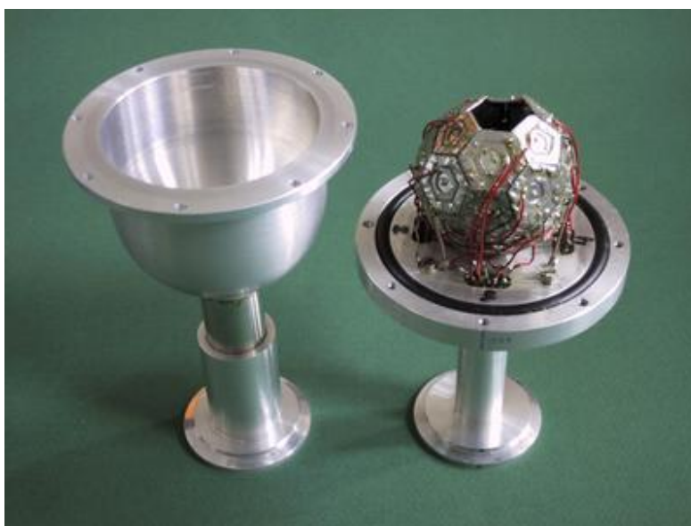
Rys. ŚLCJ-7.9: SiBall - układ detektorów krzemowych do rejestracji i identyfikacji protonów i cząstek alfa w koincydencji z detektorami germanowymi układu EAGLE (fot. A. Kordyasz)
