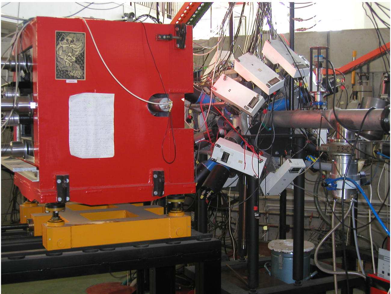
Rys. ŚLCJ-7.19: Układ do rejestracji wysokoenergetycznego promieniowania gamma JANOSIK. Na pierwszym planie widoczna jest masywna (czerwona) osłona detektora NaI (fot. J. Pluta).
