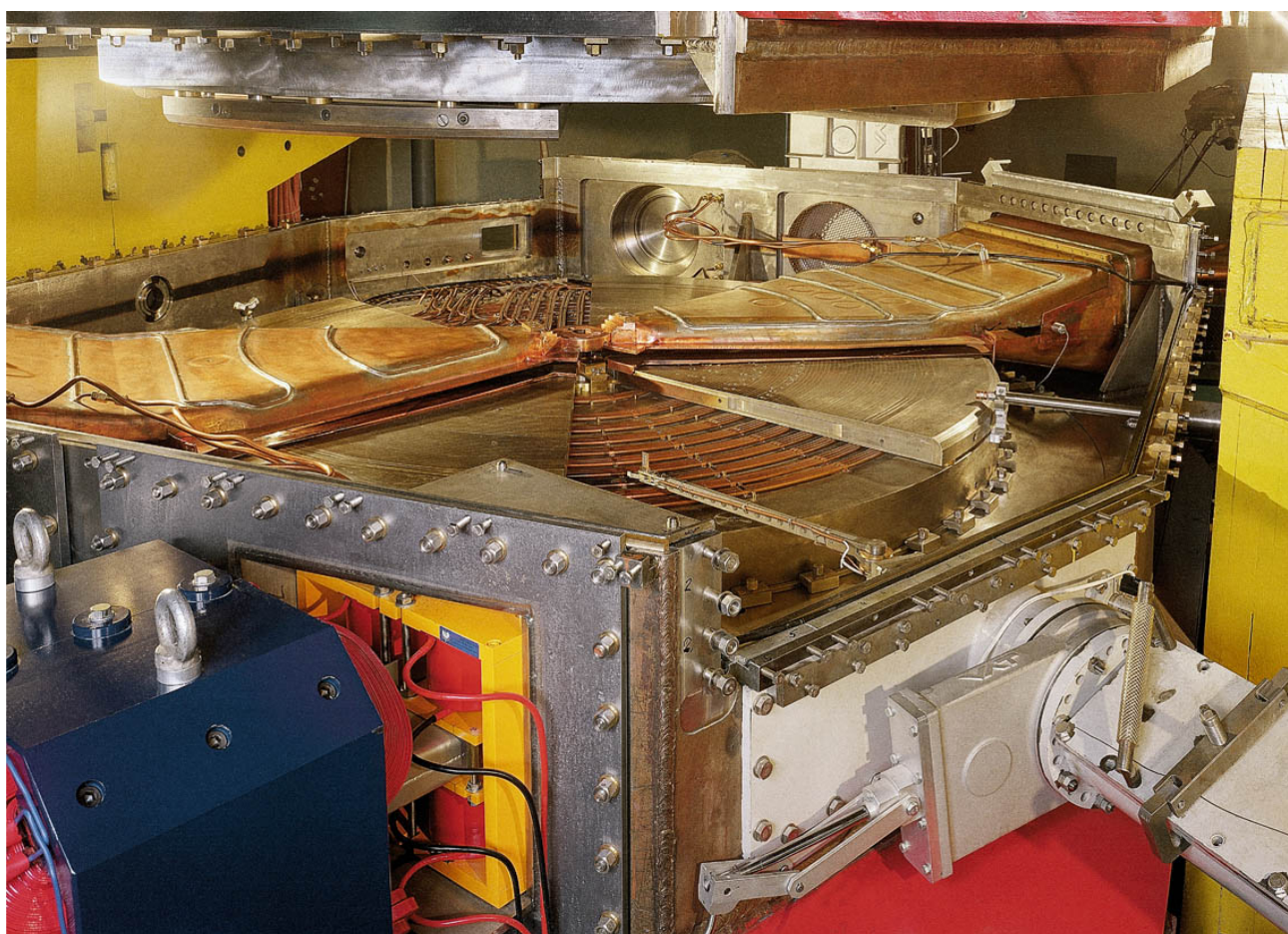
Rys. ŚLCJ-7.4: Wnętrze cyklotronu. Widoczne są dwie trójkątne elektrody przyspieszające (duanty), sektory, doliny, jak również ramię i ramka folii strippera. W lewej części zdjęcia widać pierwszy magnes kwadrupolowy (kolor niebieski) – początek jonowodu prowadzącego do stanowisk eksperymentalnych (fot. ŚLCJ).
