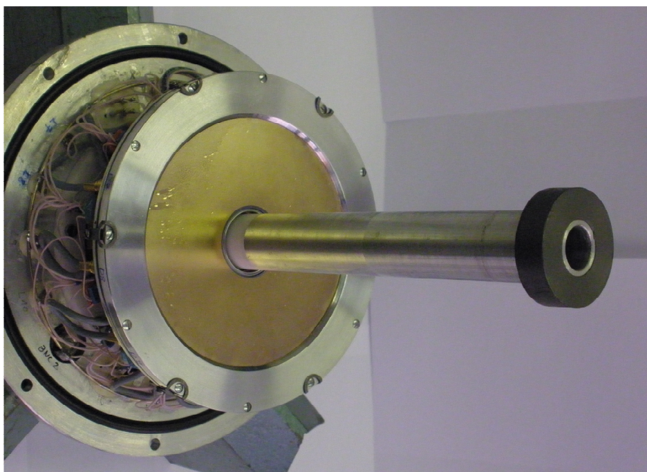
Rys. ŚLCJ-7.11: Część detekcyjna spektrometru elektronów (fot. J. Perkowski)
