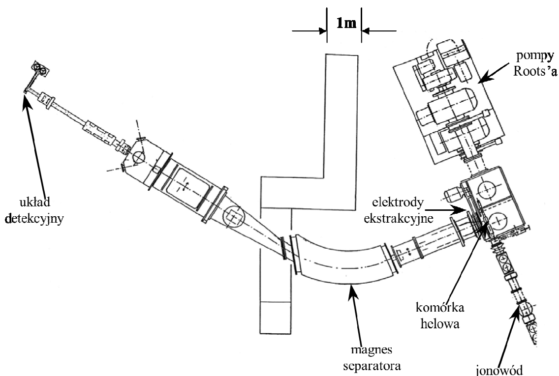
Rys. ŚLCJ-7.16: Schemat układu WIGISOL (rys. z pracy magisterskiej O.Steczkiwicz)
