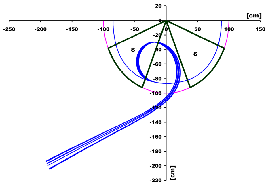
Rys. ŚLCJ-7.5: Wyprowadzenie jonów ^{14}\text{N}^{+3} przez zmianę ładunku do stanu 7+ , z promienia 83 cm. Literami „s” zaznaczono sektory, czyli obszary o wyższym polu magnetycznym (rys. J. Choiński)
