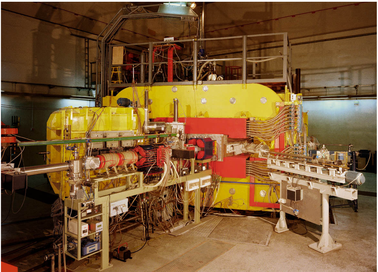
Rys. ŚLCJ-7.3: Cyklotron w ŚLCJ. Widoczny jest fragment jonowodu prowadzący jony do stanowisk eksperymentalnych (lewa strona zdjęcia) oraz układ służący do pozycjonowania folii strippera (z prawej strony) (fot. ŚLCJ)
