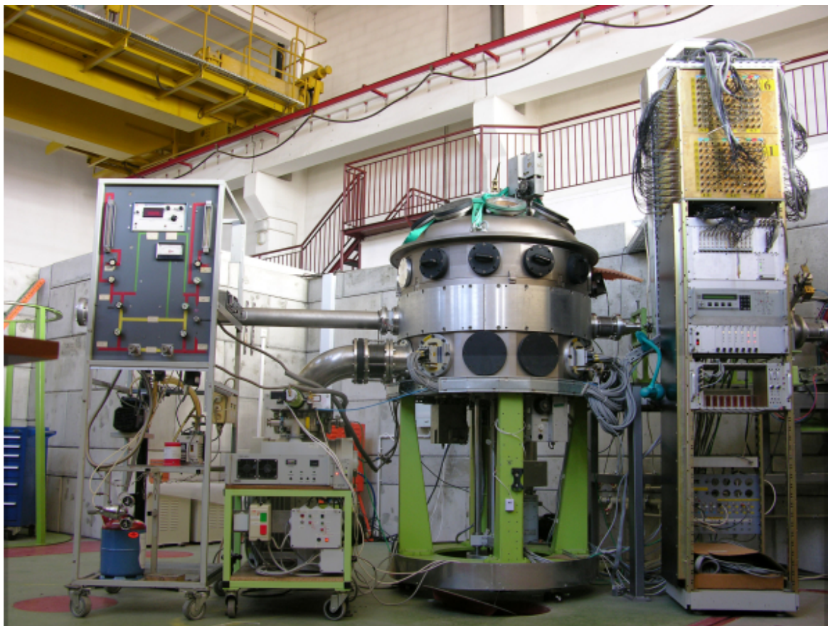
Rys. ŚLCJ-7.17: Komora ICARE do pomiarów cząstek naładowanych (fot. E. Piasecki)
