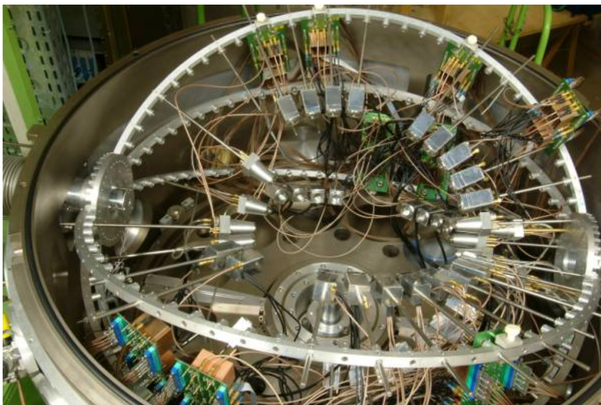
Rys. ŚLCJ-7.18: Wnętrze komory ICARE (fot. IReS Strasbourg)
