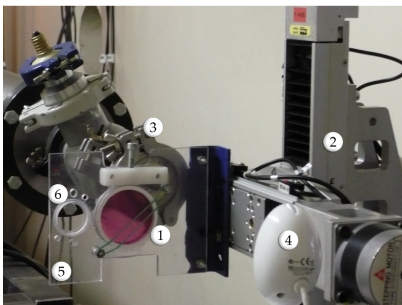
Rys. ŚLCJ-7.21: Widok układu eksperymentalnego służącego do napromieniania hodowli komórkowych wiązkami jonów. Specjalna szalka Petriego z komórkami w pożywce (nr 1) umocowana w płytce (nr 5) przytwierdzonej do stolika pomiarowego (nr 2), kamera internetowa (nr 4), zakończone folią Havarową wyjście jonowodu (nr 3), miejsce na detektor pod kątem 0 stopni względem podającej wiązki (nr 6) (fot. Z. Szepliński)
