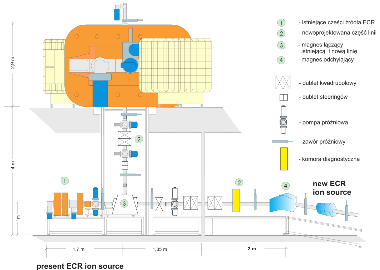
Rys. ŚLCJ-7.1: Cyklotron wraz z dwoma źródłami jonów i liniami iniekcyjnymi (rys. E. Kulczycka i I. Skrzeczanowska)
