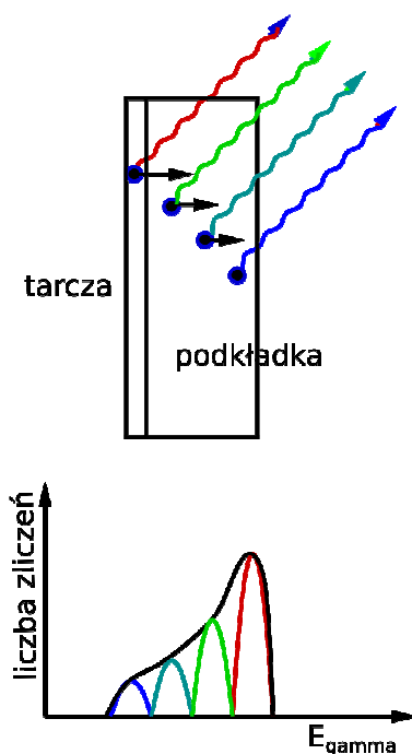
Rys. ŚLCJ-7.15: Pomiar czasu życia metodą DSAM. Kolorem czerwonym oznaczono kwanty gamma emitowane w locie, przy pełnej prędkości emitującego jądra. Kolor niebieski oznacza kwanty emitowane w spoczynku, a zielony – przy pośrednich prędkościach (rys. M.Zielińska)
