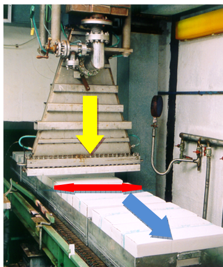
Rys. IChTJ 5.3 Widok skanera i transportera akceleratora Elektronika 10/10
