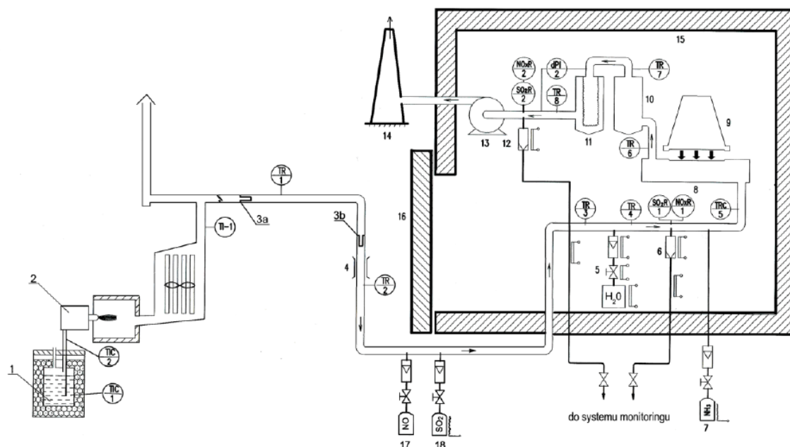
Rys. IChTJ 5.7 Schemat przepływu instalacji laboratoryjnej IChTJ do odsiarczania i odazotowania gazów odlotowych (1- zbiornik z olejem, 2- palnik olejowy, 3a- filtr do wyłapywania sadzy, 3b- filtr pyłowy, 4- kryza pomiarowa, 5- dozowanie pary wodnej, 6- pobór spalin do analizy- wlot do procesu, 7- dozowanie amoniaku, 8- komora procesowa KP, 9- akcelerator elektronów, 10- komora retencyjna, 11- filtr workowy, 12- pobór spalin do analizy- wylot z procesu, 13- wentylator wyciągowy, 14- komin, 15- ściana osłonowa, 16- drzwi osłonowe, 17- dozowanie NO, 18- dozowanie \text{SO}_2 ).
