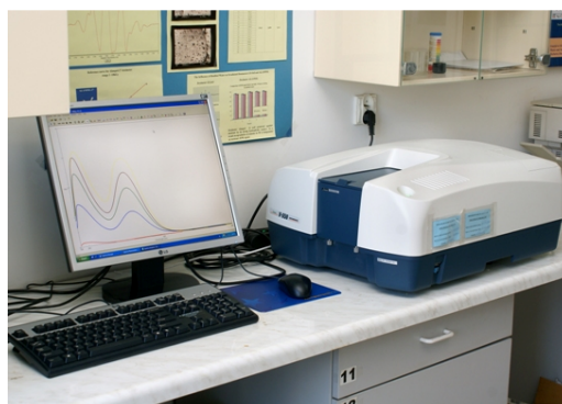
Rys. IChTJ 3.10.3 Spektrofotometr UV-Vis JASCO V-650
