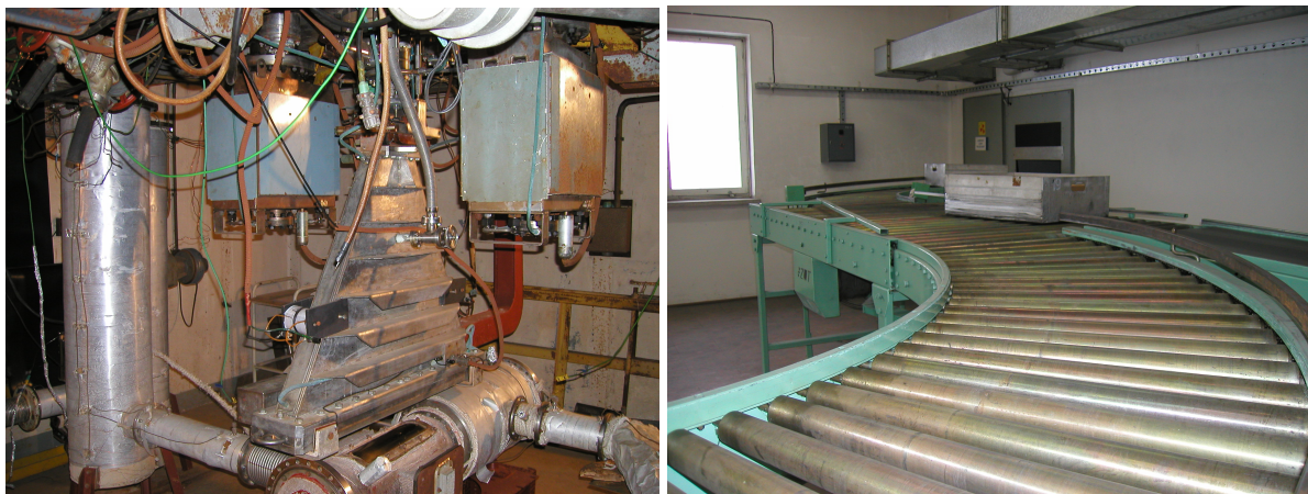
Rys. IChTJ 3.2.1 Akcelerator elektronów
