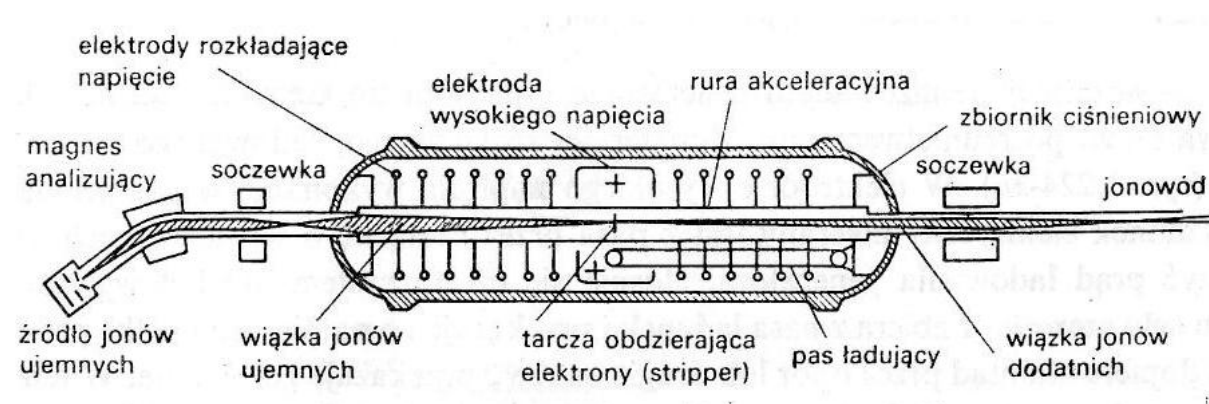
Rys. 2.2.13. Schemat akceleratora typu „Tandem” [1]
