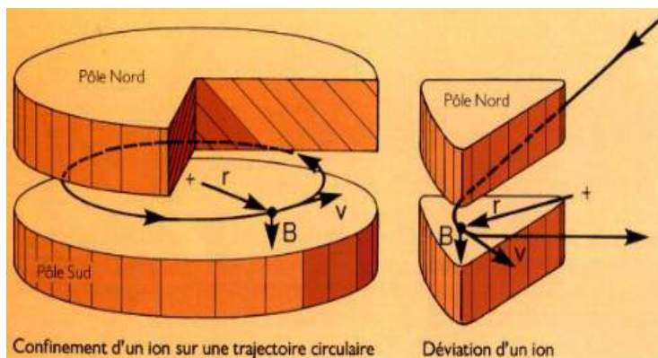
Rys.2.2.18 Nabiegunniki magnesu cyklotronu
