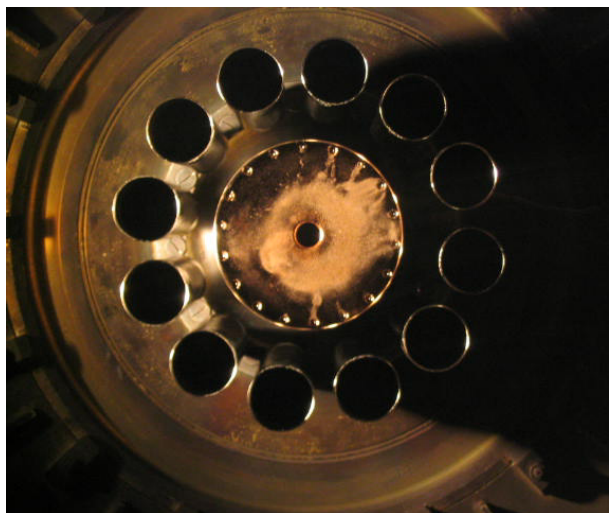
Rys. IFPiLM-7. Wnętrze komory PF-1000 z widocznymi elektrodami wewnętrzną i zewnętrzną.
