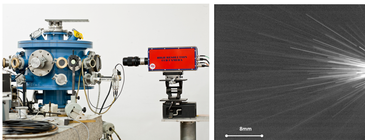
Rys. IFPiLM-13. Stanowisko eksperymentalne do badań pyłów powstających w wyniku oddziaływania impulsów laserowych z tarczami z widoczną po prawej stronie kamerą CCD wraz z przykładowym zdjęciem zarejestrowanym w eksperymencie z tarczą z tokamka TEXTOR.
