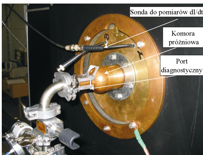
Rys. IFPiLM-9. Mobilne urządzenie PF-6 w IFPiLM z widoczną po prawej stronie komorą próżniową
