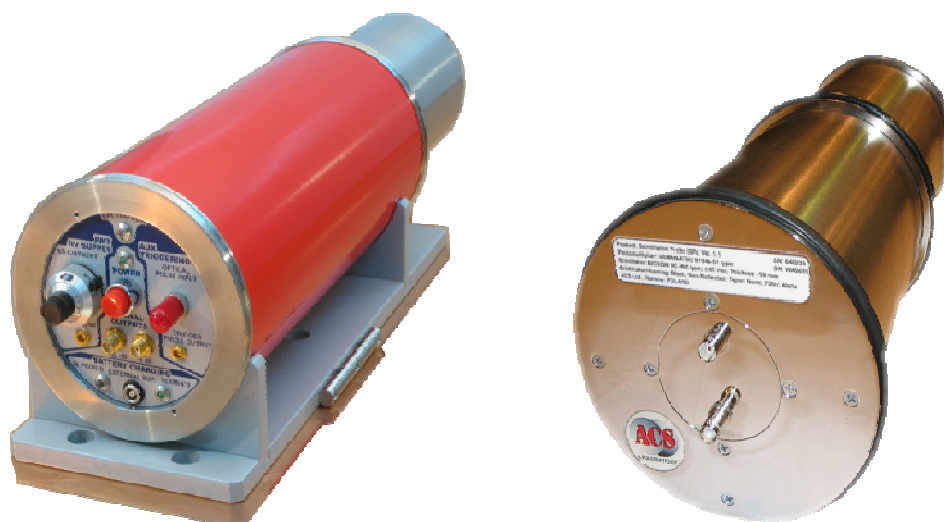
Rys. IFPiLM-8. Scyntylniki do pomiarów neutronowych: MCP-PMT i ultraszybki BC-422Q (BICRON) scyntylnik plastikowy (po lewej) oraz klasyczny PMT i szybki BC-408 (BICRON) scyntylnik plastikowy (po prawej)
