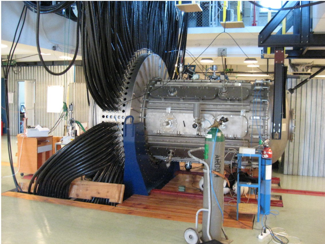
Rys. IFPiLM-6. Urządzenie Plasma-Focus PF-1000 w IFPiLM
