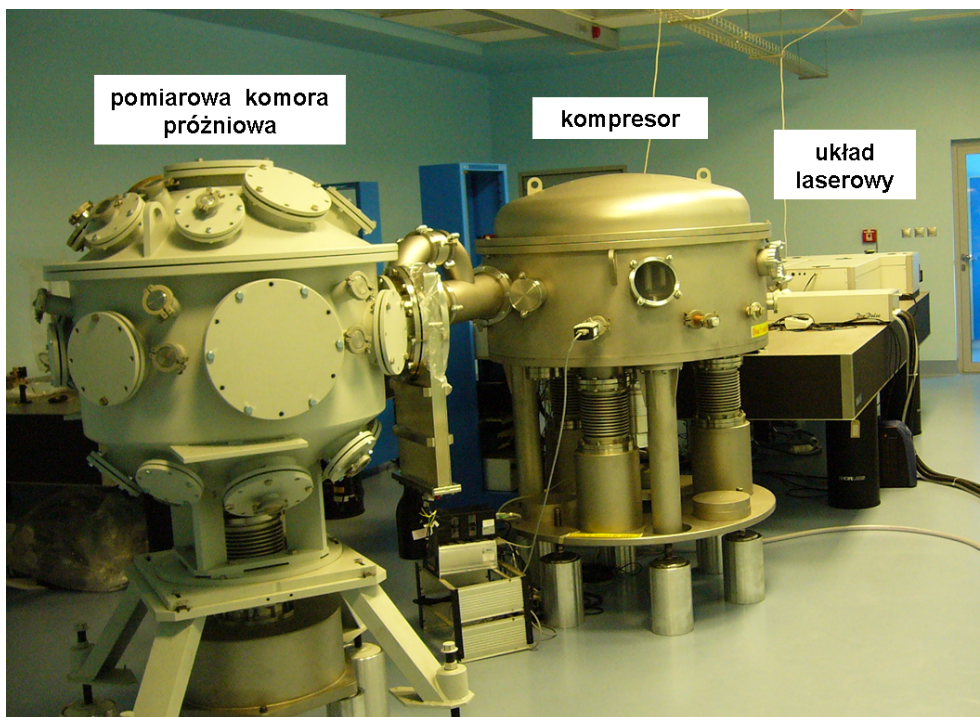
Rys. IFPiLM-10. Układ lasera femtosekundowego wielkiej mocy zlokalizowanego w laboratorium Oddziału Plazmy Wytwarzanej Laserem w IFPiLM
