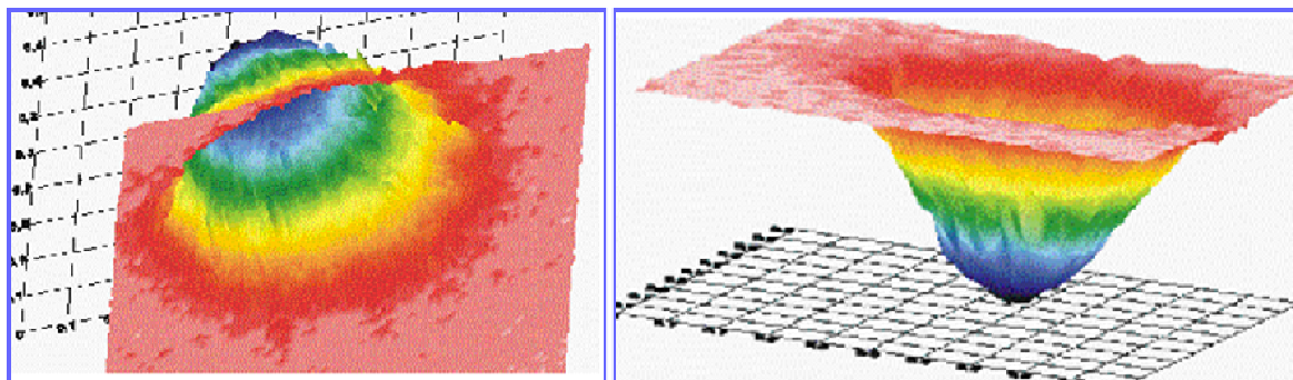
Rys. IFPiLM-14. Przykład zmierzonych profilometrem kraterów po oddziaływaniu lasera Nd:YAG z tarczą grafitową dla dwóch gęstości mocy: P = 9.4\text{MW}/\text{cm}^2 , gdzie głębokość krateru wyniosła 240\text{ }\mu\text{m} (po lewej) oraz P = 8.3\text{MW}/\text{cm}^2 , gdzie głębokość krateru wyniosła 210\text{ }\mu\text{m} (po prawej).
