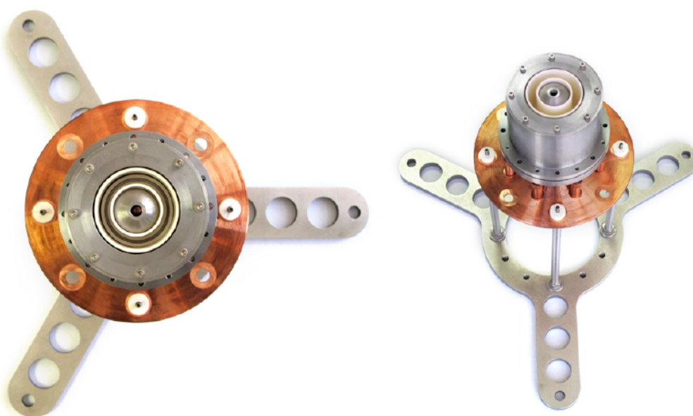
Rys. IFPiLM-4. Zdjęcia kryptonowego silnika Halla wykonanego w IFPiLM ze zdemonstrowaną katodą [J. Kurzyna et al. IEPC-2011-221, 2011]
