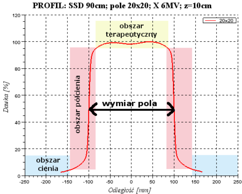
Rys. 5. Przykładowy profil pola 20cm x 20cm na głębokości 10 cm, dla wiązki fotonów o energii 6MV.
