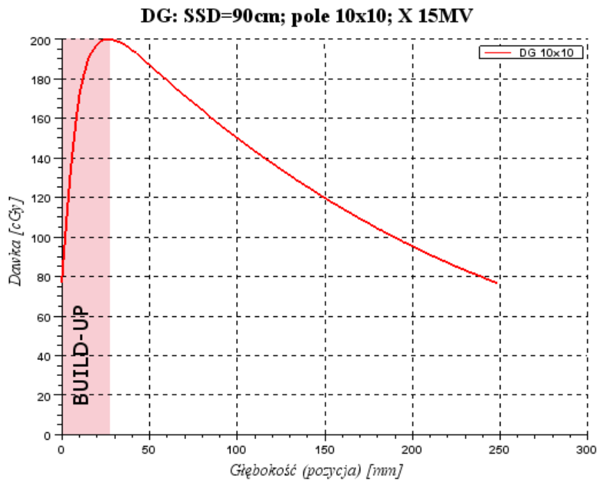
Rys. 3. dla pola 10cm x 10cm, wiązka fotonowa o energii 15MV.
