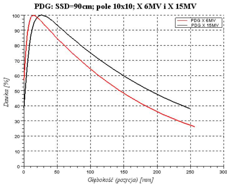
Rys. 4. Porównanie dla wiązek fotonowych o energii 6MV oraz 15MV, pole 10cm x 10cm, SSD = 90 cm.
