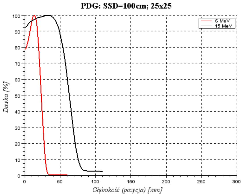
Rys 16. Porównanie dla wiązek elektronów o energiach: 6MeV i 15MeV, pole 25cm x 25cm, SSD = 100 cm.
