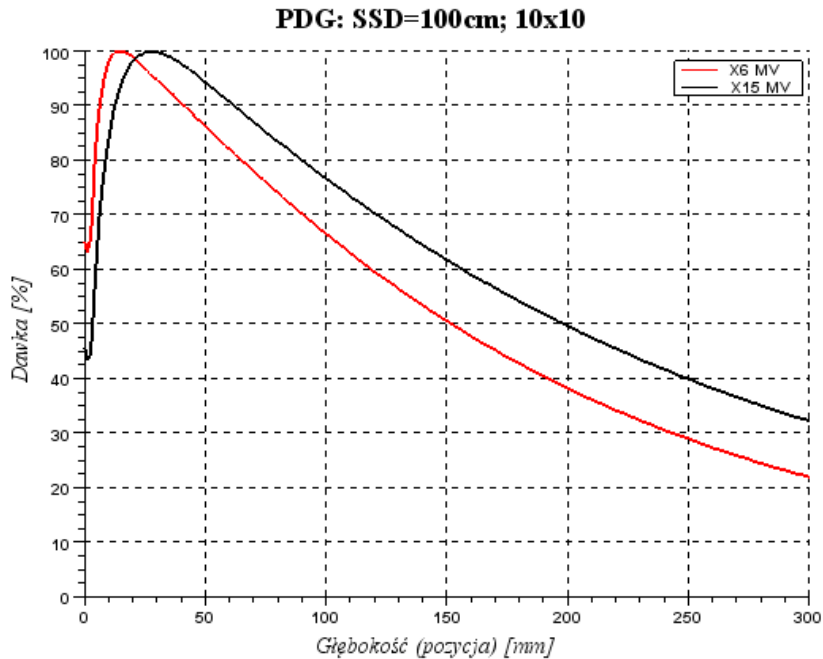
Rys 15. Krzywe dla wiązek fotonowych o energii 6MV i 15MV, pole 10cm x 10cm, SSD = 100 cm.
