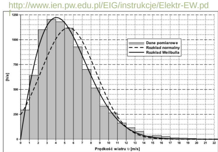
Rys. 2. Histogram prędkości wiatru dla Leby i zastosowanie rozkładu normalnego oraz Weibulla.
