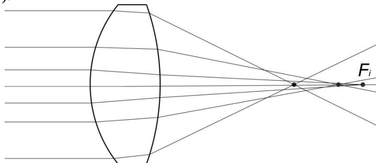
Rys. 7 – Aberracja sferyczna.
