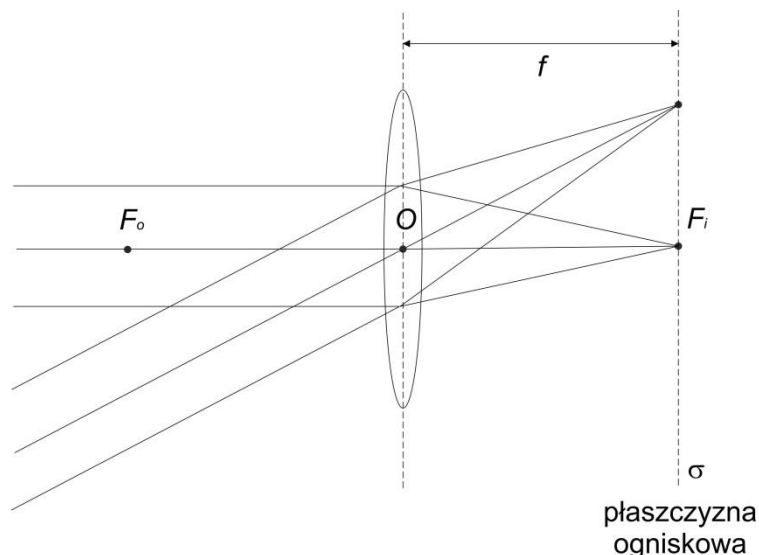
Rys. 2 – Ogniskowanie idealnej soczewki cienkiej.
