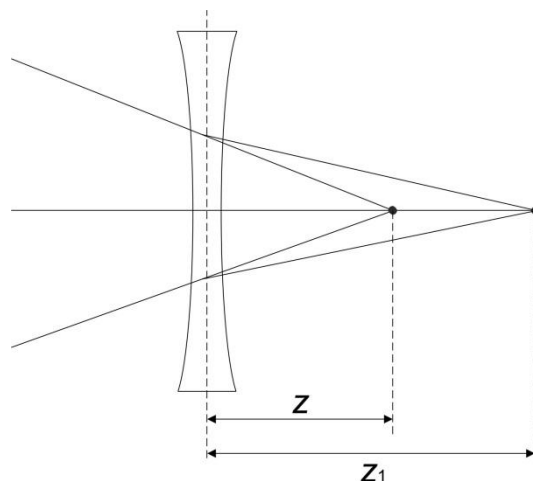
Rys. 11 – Wyznaczanie ogniska soczewki rozpraszającej.
