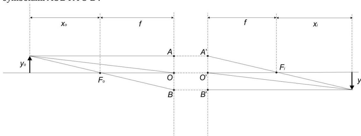
Rys. 6 – Płaszczyzny główne.
