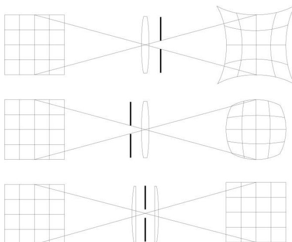
Rys. 10 – Dystorsja.
