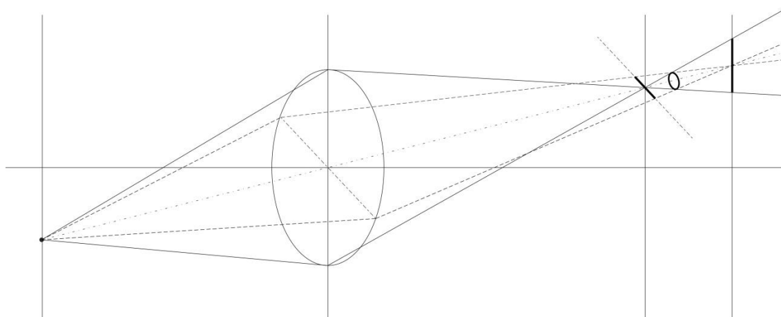
Rys. 9 – Astygmatyzm.
