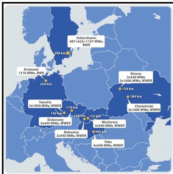
Rys. CLOR-4. Elektrownie jądrowe (wraz z pracującymi w nich reaktorami) w odległościach nie większych niż 300 km od granic naszego kraju.
