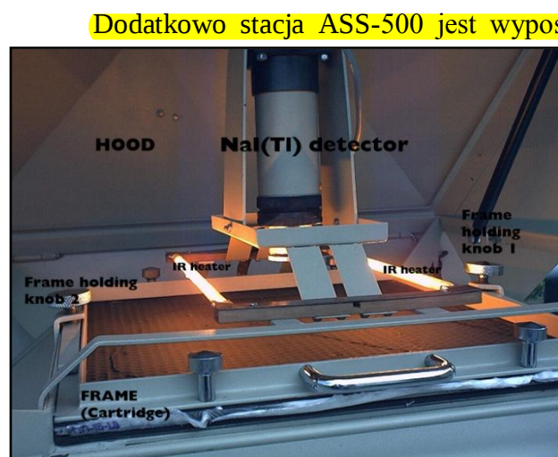
Rys. CLOR-6. Sonda scyntylacyjna NaI(Tl) umieszczona nad filtrem powietrza w stacji ASS-500 (element systemu on-line)
